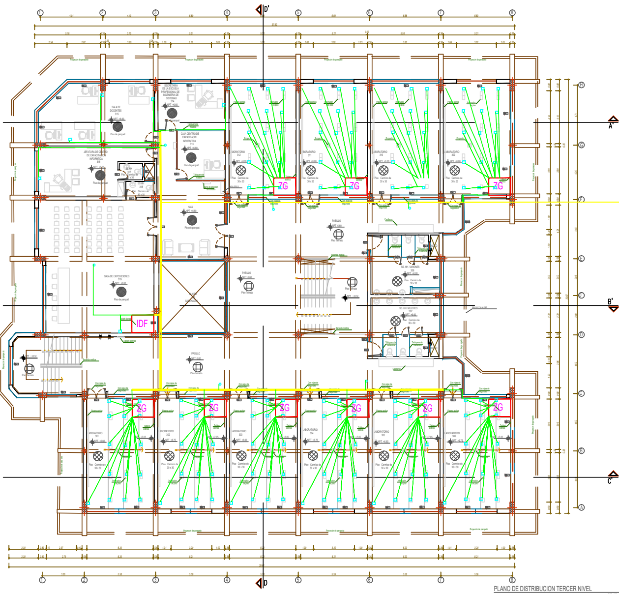
PLANO DE DISTRIBUCION TERCER NIVEL
